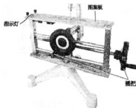
图 3-4 BD-II-302 型双手调节器
