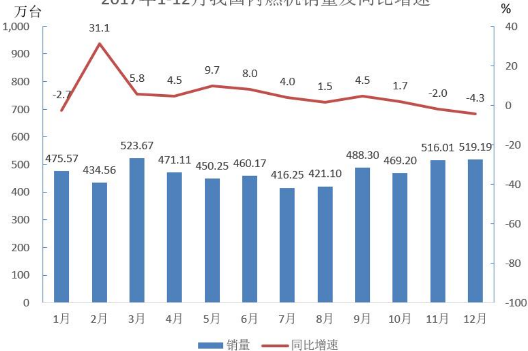
2017年1-12月我国内燃机销量及同比增速
